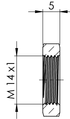
Ansicht / view A-A
