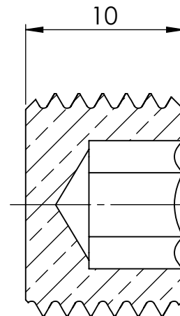
SCHNITT A-A
