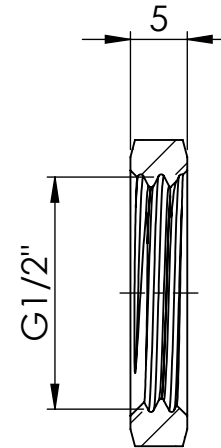
SCHNITT A-A
