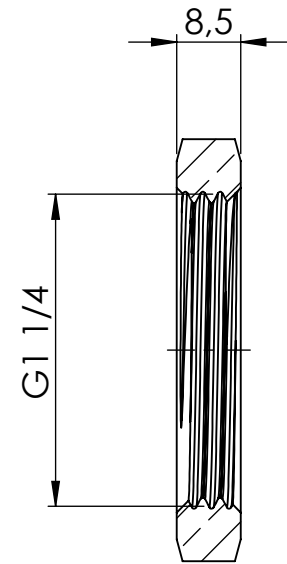
SCHNITT A-A
